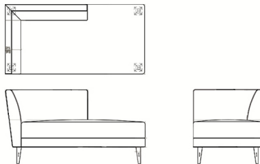
► PC222 CHAISE LOUNGE 60"W X 30"D X 32"H
